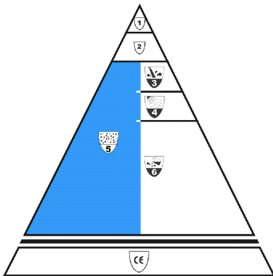
EN 14605:2005 Type 3 Vloeistofdichte kleding
